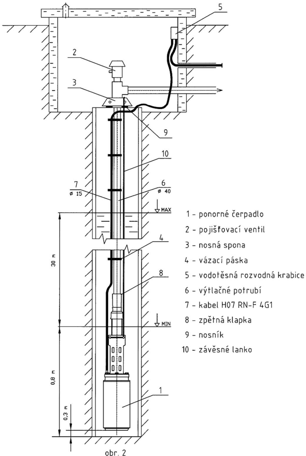
Hlavní části čerpačícího zařízení a montáž čerpadla do vrtu
